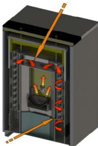
Турболатори по димна страна с ръчно почистване без нужда от отваряне на горивната камера
