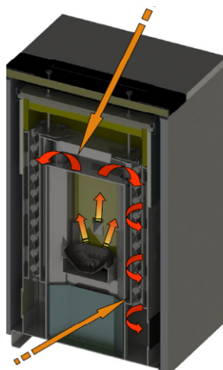
Турболатори по димна страна с ръчно почистване без нужда от отваряне на горивната камера
